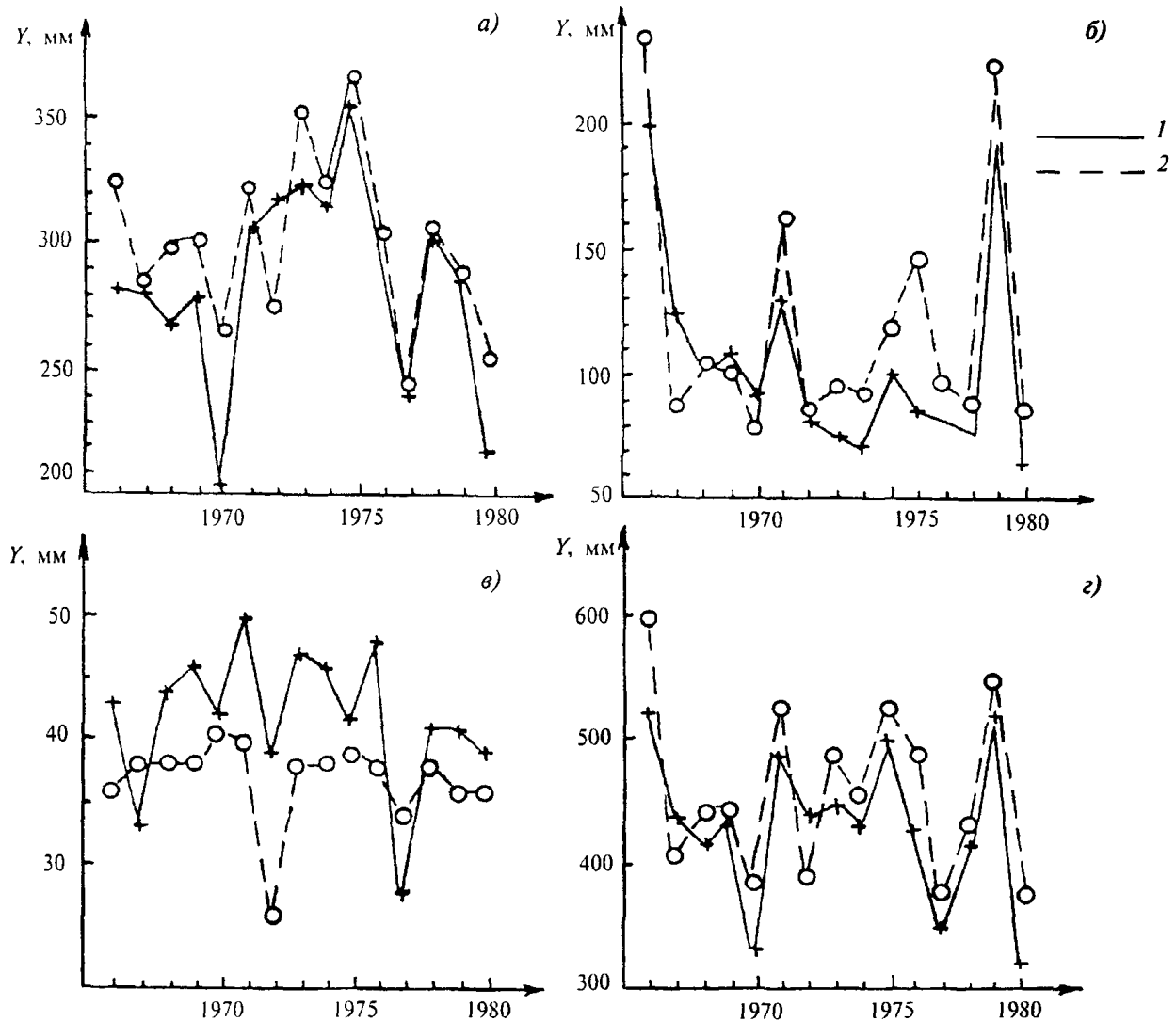
а) — весеннее половодье; б) — летне-осенний сезон; в) — сезон зимней межени; з) — годового стока Рисунок А.5 — Сравнение фактических (1) и рассчитанных (2) слоев стока р. Вага — с. Усть-Сюма
