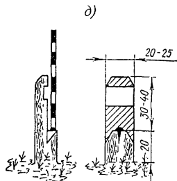
Рис. 4.1. Типы знаков долговременного закрепления пунктов съёмочного обоснования
