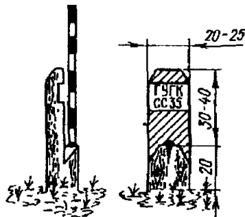
Рис. 44. Тип знака долго- временного закрепления пунктов съемочных сетей в залесяных районах
