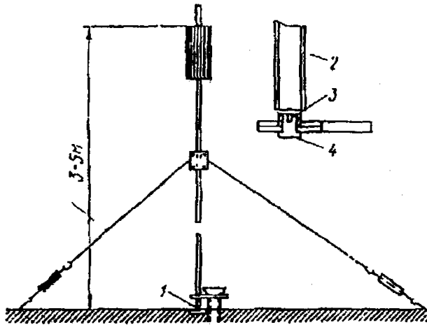
Рис. 31. Съёмная металлическая точка с визирным цилиндром 1 — центр пункта; 2 — веха, 3 — отверстие (центр пункта); 4 — болт
