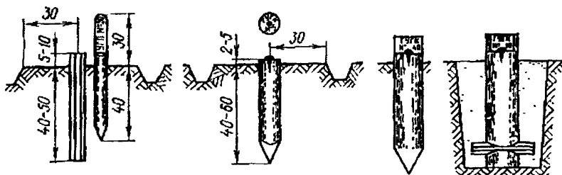
Рис. 45 Металлическая труба, кованый гвоздь со сторожкой
