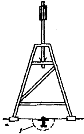
Рис. 30. Пирамидаштатив со съёмной визирной целью 1 — марка триангуляционная
