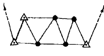
Рис. 23 Цепочка треугольников между стороной и пунктом
