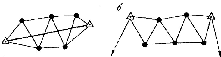
Рис. 24 Цепочки треугольников между двумя пунктами
