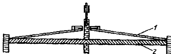
Рис. 29. Тур со съемной визирной целью 1 — крышка; 2 — перекрытие (балка)
